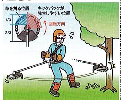
一般社団法人日本農業機械工業会 「刈払機の正しい使い方」より
